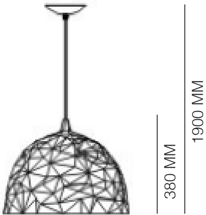
Ø 500 MM
